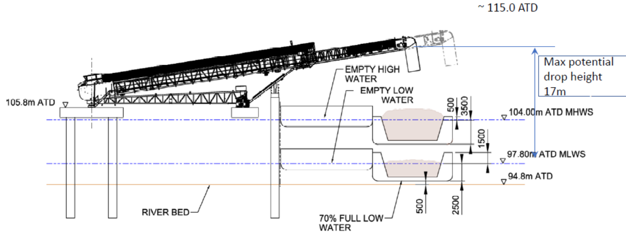
SECTION A-A Scale: 500
